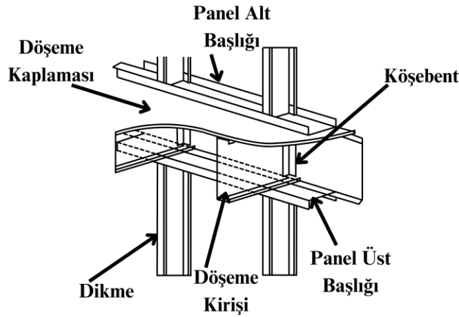
Şekil 7.2: Platform iskelet
