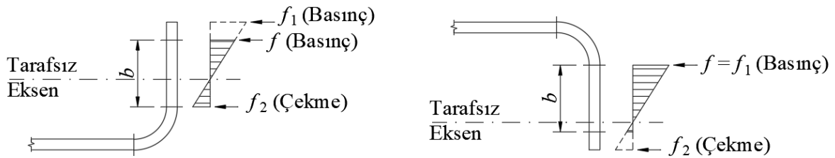
(a) Basınç etkisindeki desteklenmeyen kenar
