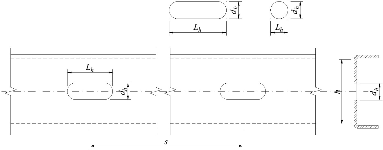
Şekil 10.1: Boşluk geometrisi
