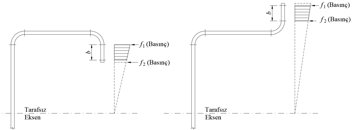
(a) İç bükey kenar rijitleştirici
