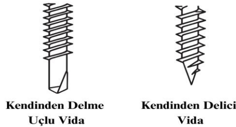
Şekil 8.1: Yaygın Kullanılan Vida Uç Tipleri
