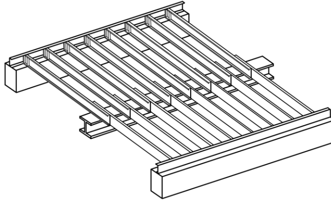
Şekil 9.1: Temel Sistemi (Örnek)
