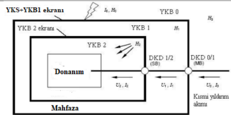
Şekil 7.5a- Hacimsel ekranlama ve koordineli DKD sistemi kullanan YEKS – Donanım, iletilen darbelere karşı korunmuştur ( U_2 \ll U_0 ve I_2 \ll I_0 ) ve ışımla yayılan manyetik alanlara karşı da korunmuştur ( H_2 \ll H_0 )
