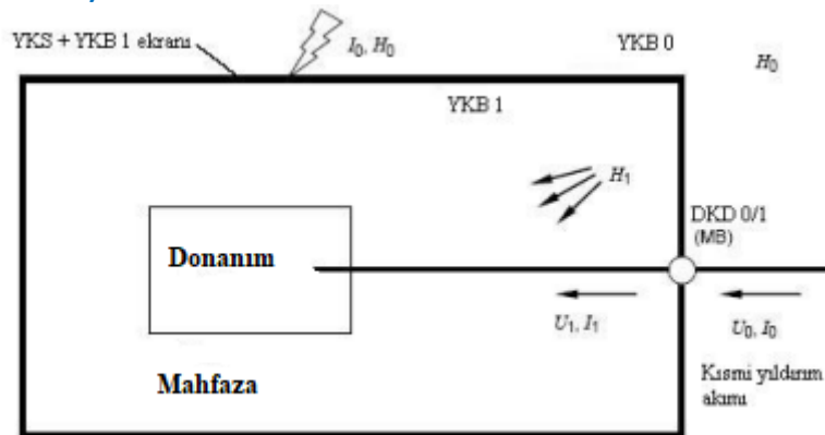
Şekil 7.5b-YKB 1'in hacimsel ekranını ve YKB 1 girişinde DKD korumasını kullanan YEKS – Donanım, iletilen darbelere karşı korunmuştur ( U_1 < U_0 ve I_1 < I_0 ) ve ısıma ile yayılan manyetik alanlara karşı da korunmuştur ( H_1 < H_0 )
