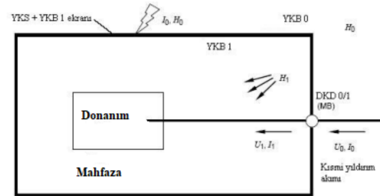
Şekil 7.5b-YKB 1'in hacimsel ekranımı ve YKB 1 girişinde DKD korumasını kullanan YEKS – Donanım, iletilen darbelere karşı korunmuştur ( U_1 < U_0 ve I_1 < I_0 ) ve ışınlımla yayılan manyetik alanlara karşı da korunmuştur ( H_1 < H_0 )
